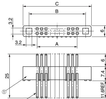
Wire wrapping type HKP-( )M4W
