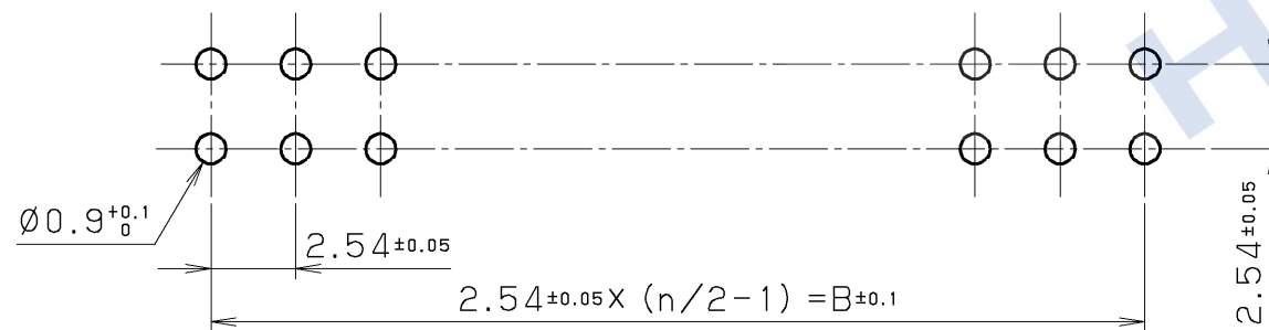
基板参考寸法 (4/1) RECOMMEND BOARD
