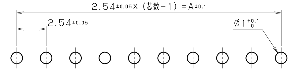
推奨基板穴径寸法
