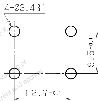
基板取付穴加工図
