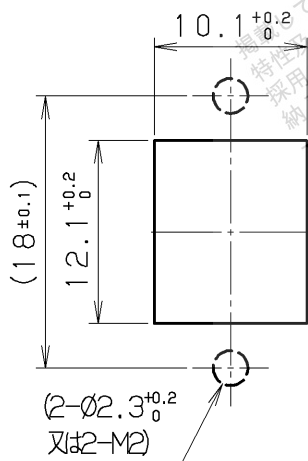
取付穴寸法図
