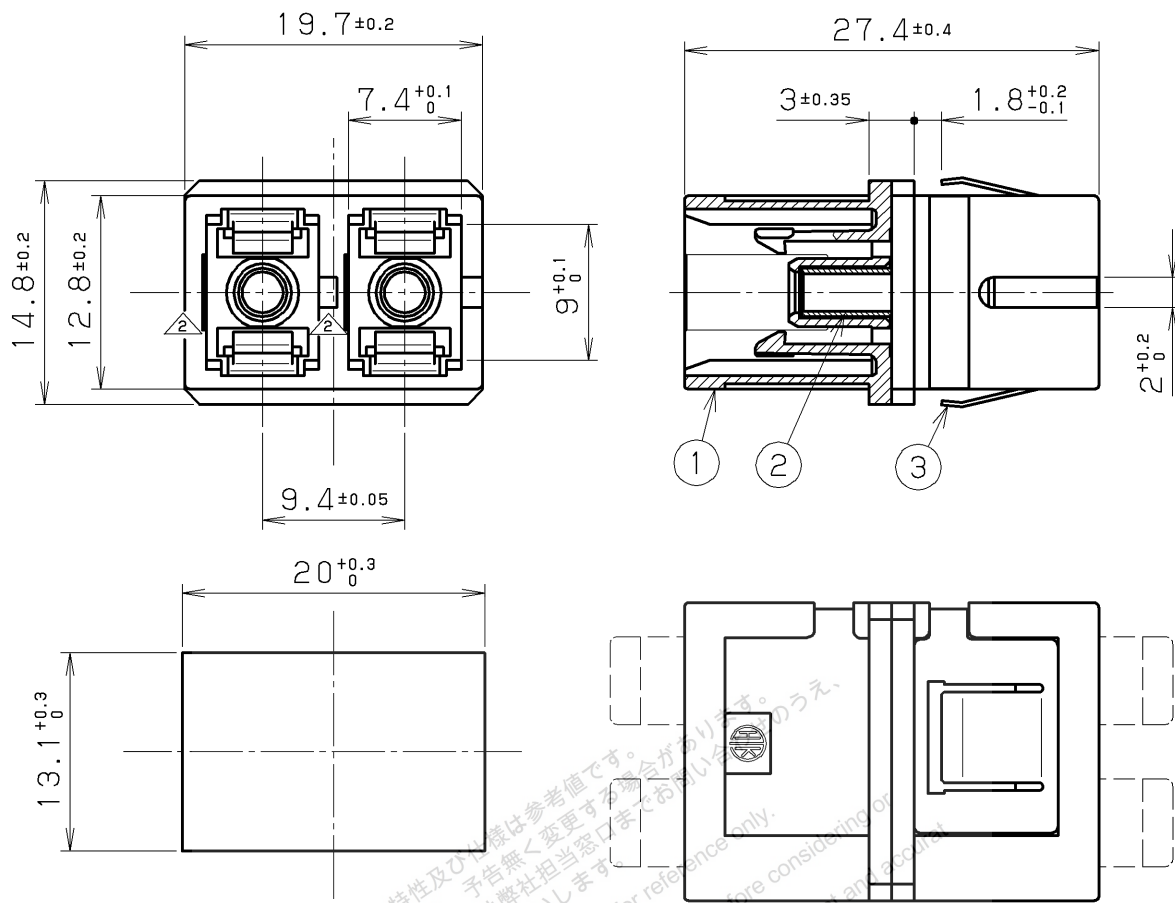
△ 取付穴寸法図 (基板厚: t=1.6)
