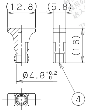
④キャップ (S=1/1)
