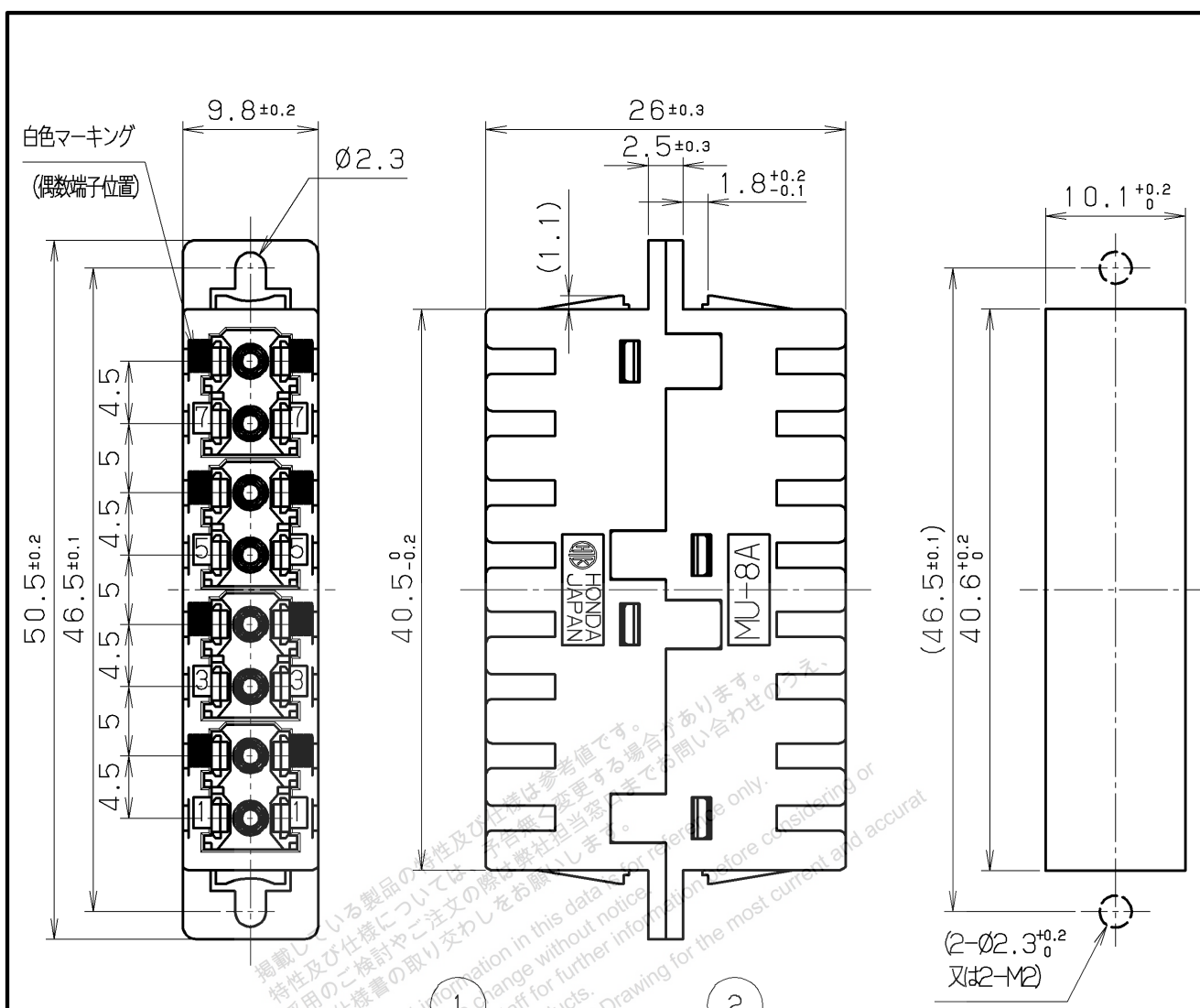
取付寸法図
