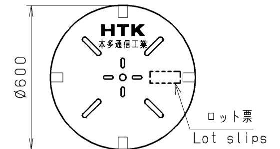
リール形状図 Reel Style and Dimensions
