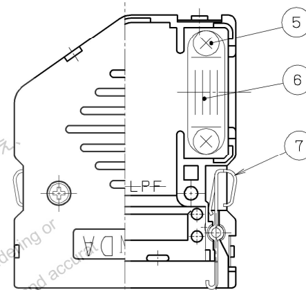
ケース内部詳細図
