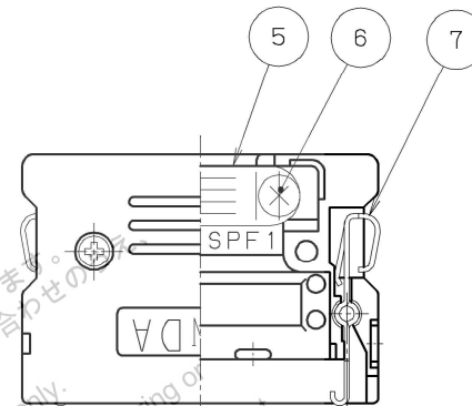
ケース内部詳細図
