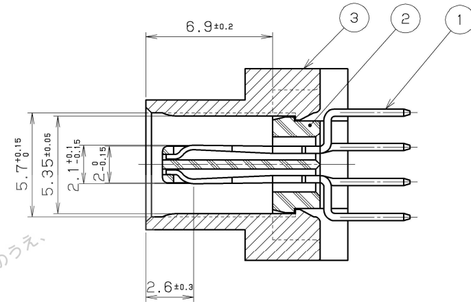
X-X断面矢視 (5/1)
