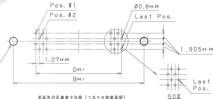
基板取付孔参考寸法図 (コネクタ実装面図)
