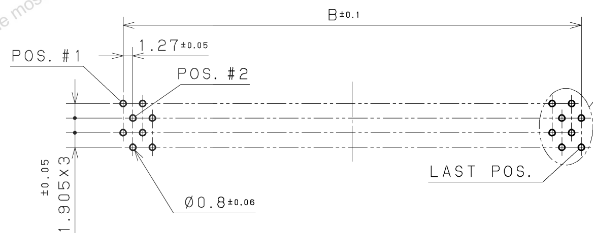
基板取付け寸法図 実装面側
