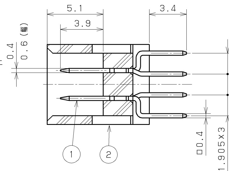
コンタクト形状図
