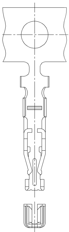
A 矢視
